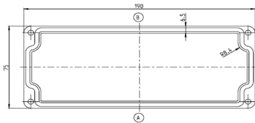
Unterteil
