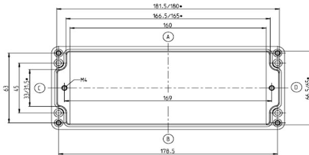
Unterteil
